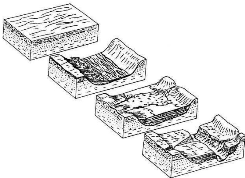
Figure 2.9. Venosa Basin. The evolution of the landscape (after Soprintendenza Speciale al Museo Nazionale Preistorico Etnografico “L. Pigorini” 1991).
