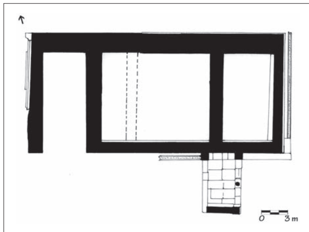
10.15. Plan. Building ABCD, Hagia Triada. After Di Vita and La Regina 1984, fig. 230.
