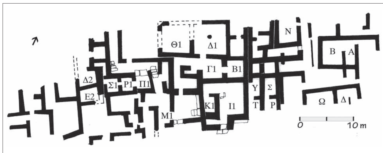
11.12. Plan. Khondro Viannou. After L. Platon 1997, fig. 4.
