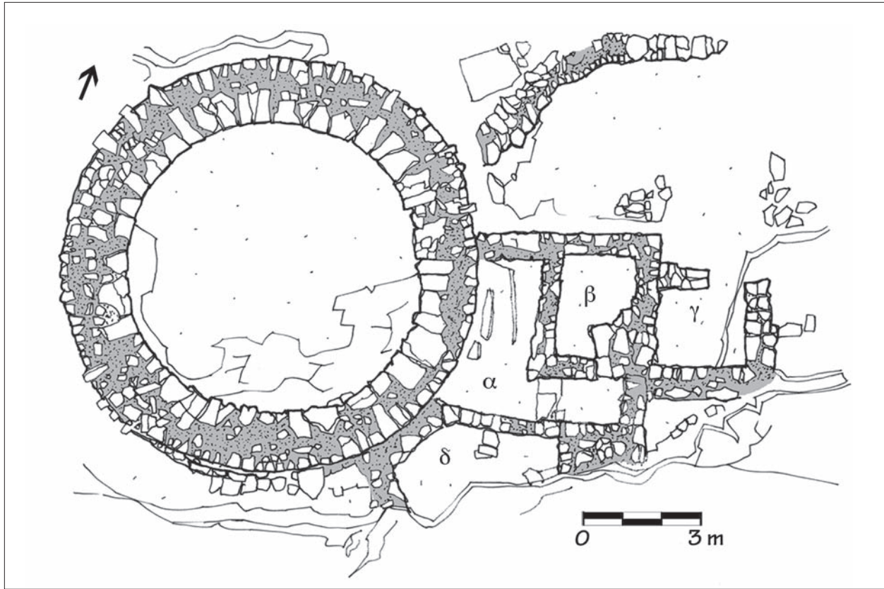
5.11. Plan. Tholos Tomb, Kamilari. After Di Vita and La Regina 1984, fig. 309.
