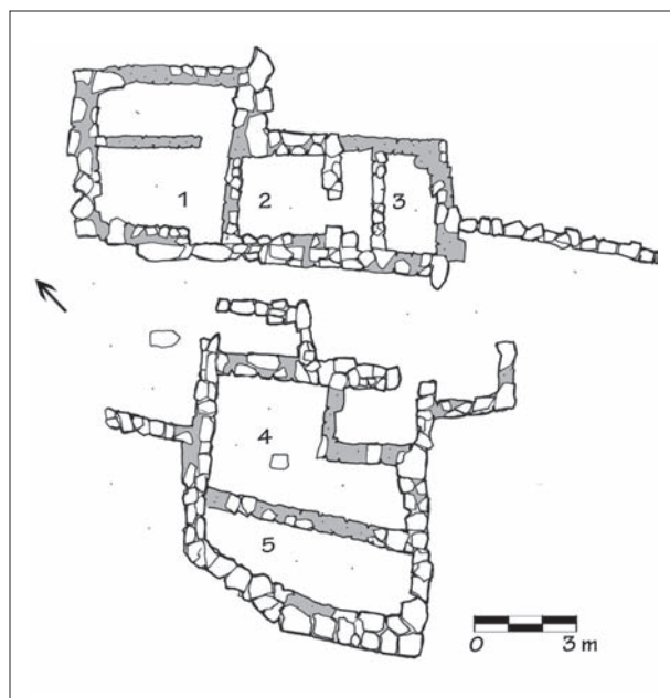
4.10. Plan. Quartier Theta. After H. and M. van Effenterre 1976, pl. 30.
