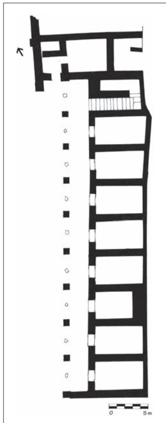
11.5. Plan. Stoà del Mercato. After Di Vita and La Regina 1984, fig. 230.
