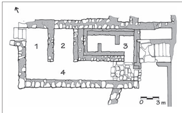
6.19. Plan. Sanctuaire des Cornes, Malia. After Daux 1957, fig. 15 bis.
