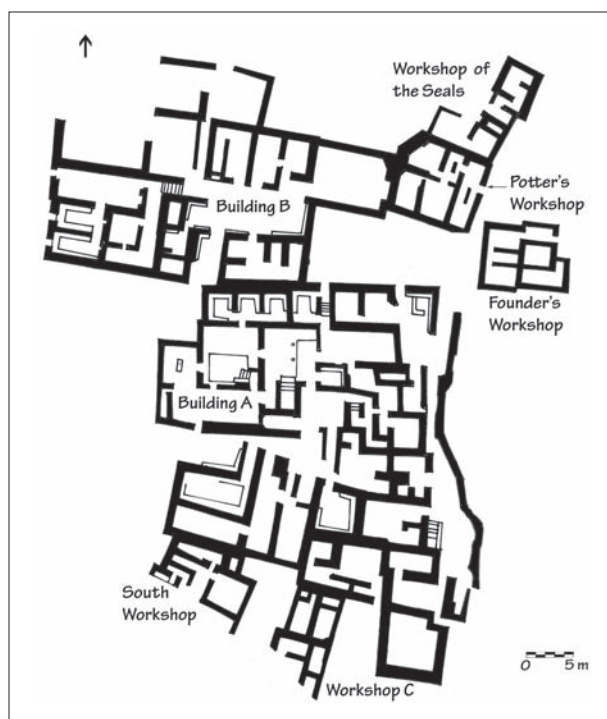
6.15. Plan. Quartier Mu, Malia. After Poursat 1992, plan.
