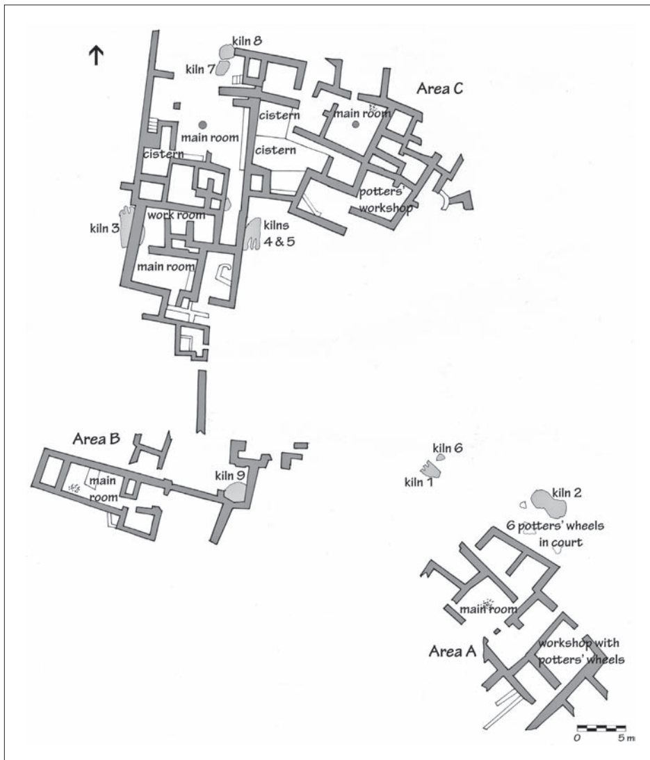
11.16. Plan. Kato Gouves. After Vallianou 1997, pl. CXXIV.
