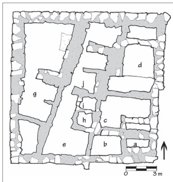
4.11. Plan. Maison B, Malia. After Demargne and Gallet de Santerre 1953, pl. LXI.
