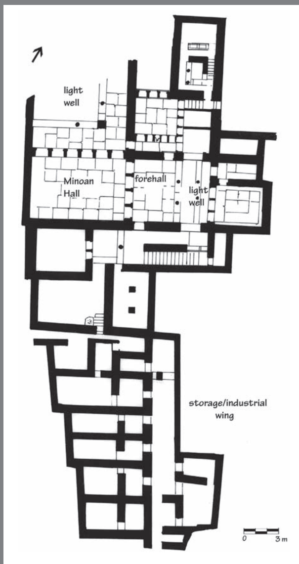
9.22. Plan. House A, Haghia Triada. After Di Vita and La Regina 1984, fig. 230.
