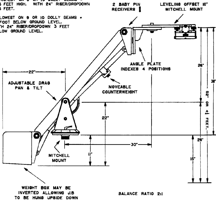
Figure 10.24a Fisher Jib, Model 20 (J. L. Fisher Mfg.).
