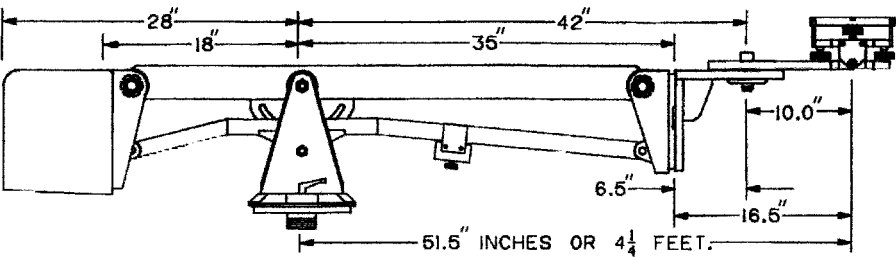
Figure 10.24b Fisher Jib, Model 20 (J. L. Fisher Mfg.).
