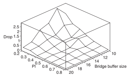
(d) Bridge from P2 to P1, M_b = 12 .
