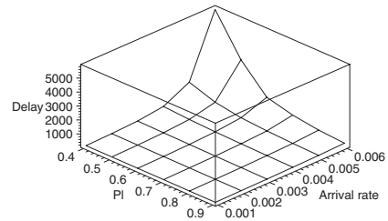
(d) Interior piconets, M_s = 5 .
