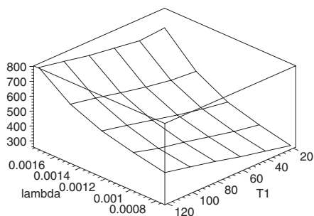
(d) Exhaustive polling, simulation results.
